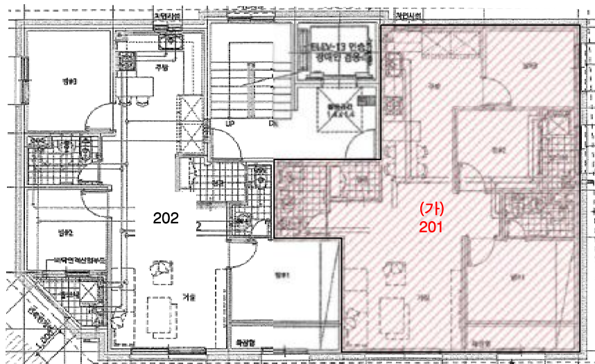
[더머뎀 제비동 제2층 호별배치도 및 제201호 내부구조도]
